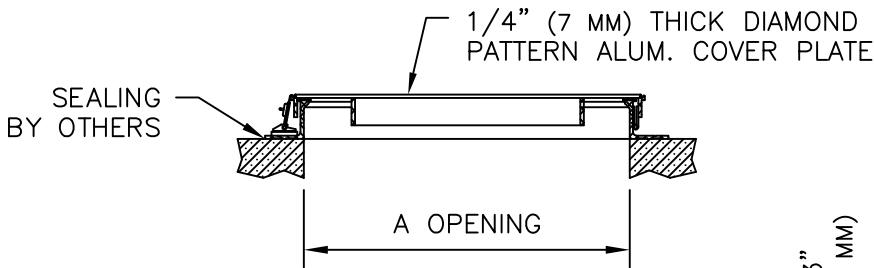
SECTION A-A
